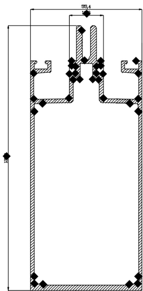
83036-00 2,400 Kg/m
