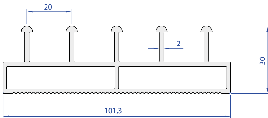
75352-00 1,643 Kg/m
