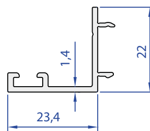
85010-00 0,226 Kg/m
