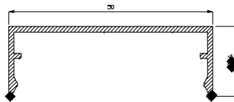
83031-00 0,310 Kg/m
