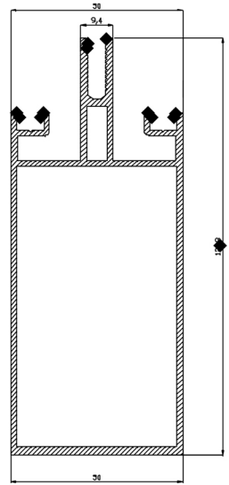
83029-00 2,062 Kg/m
