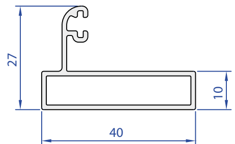
75400-00 0,413 Kg/m
