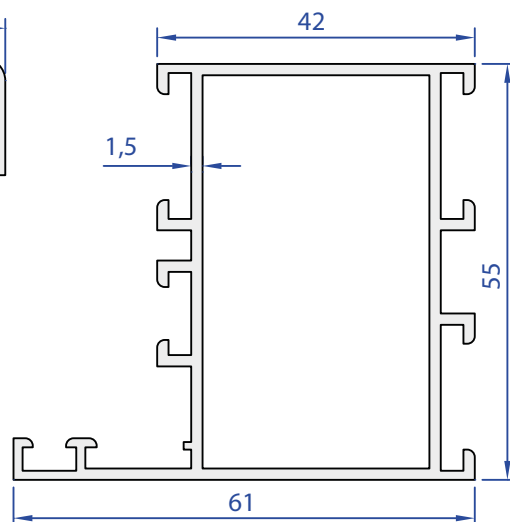
81001-00 1,033 kg/m
