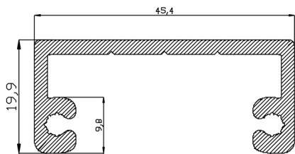
83033-00 0,686 Kg/m
