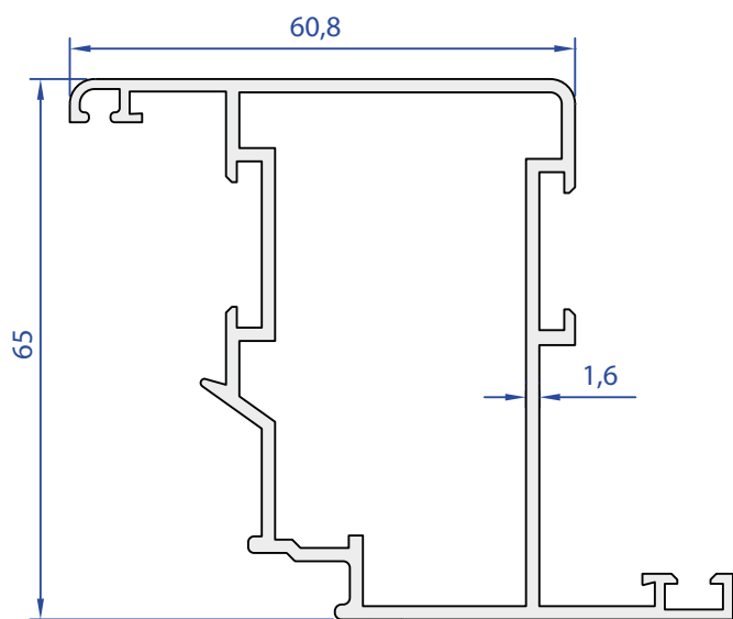
81015-00 1,247 Kg/m
