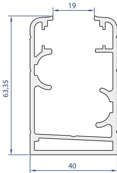
75472-00 1,439 Kg/m
