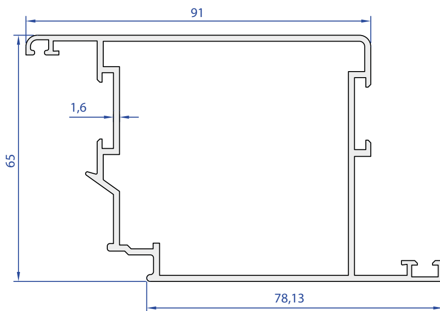
81011-00 1,509 Kg/m
