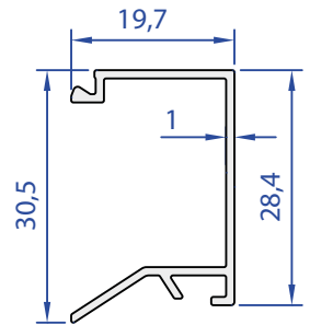
80010-00 0,208 kg/m
