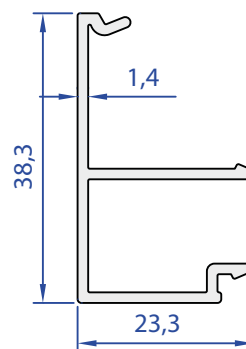
81006-00 0,354 kg/m
