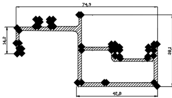
83027-00 1,051 Kg/m
