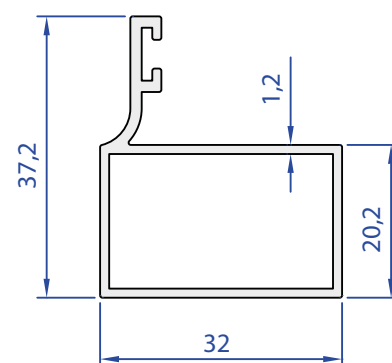
75537-00 0,428 Kg/m
