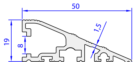
05429-00 0,602 kg/m
