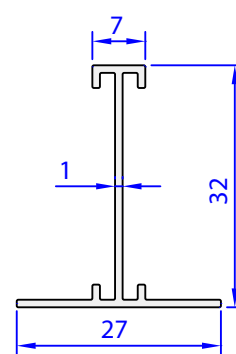
05161-00 0,195 kg/m
