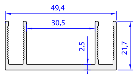
05264-00 0,593 kg/m
