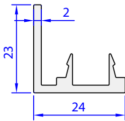
06154-00 0,329 kg/m
