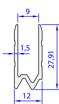
05147-00 0,263 kg/m
