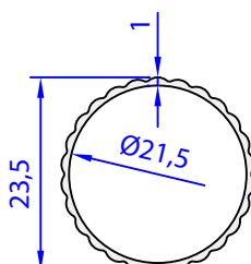
05200-00 0,158 kg/m
