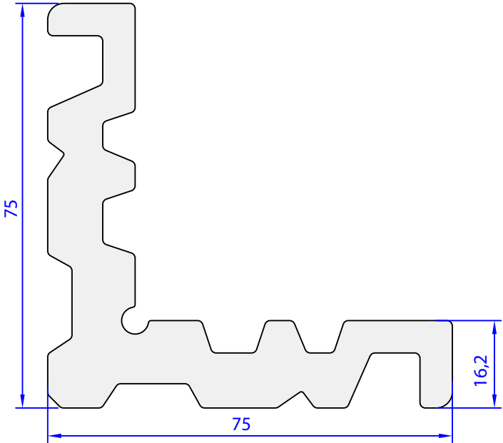
05582-00 4,186 kg/m
