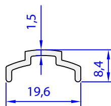
05061-00 0,121 kg/m
