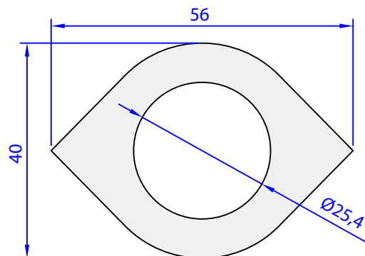
05041-00 2,476 kg/m
