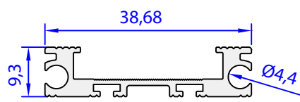
05560-00 0,322 kg/m
