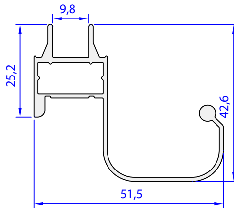
05241-00 0,540 kg/m
