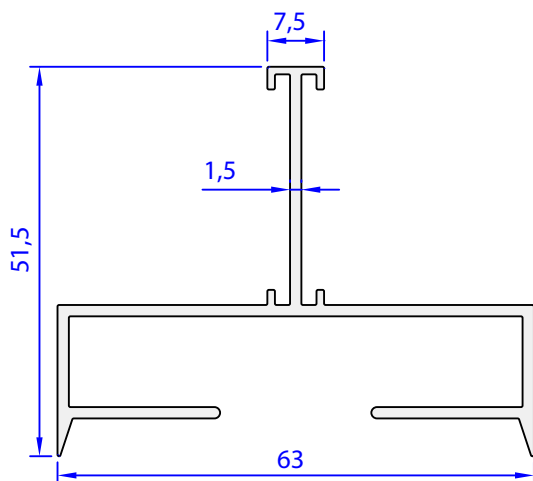
05160-00 0,725 kg/m
