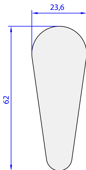
05094-00 2,839 kg/m
