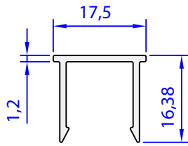
06155-00 0,154 kg/m
