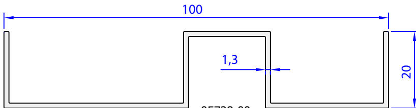
05728-00 0,615 Kg/m
