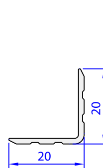
05563-00 0,138 kg/m
