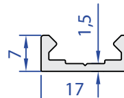
70007-00 0,140 kg/m
