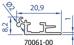
70061-00 0,123 kg/m
