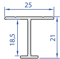
60363-00 0,191 Kg/m
