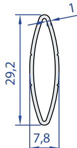
60001-00 0,161 kg/m
