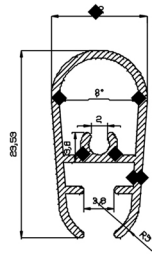
60790-00 0,197 Kg/m
