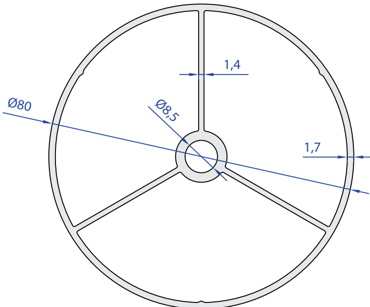
05918-00 1,732 Kg/m
