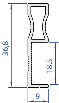
60365-00 0,269 Kg/m
