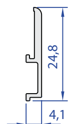
60044-00 0,118 kg/m
