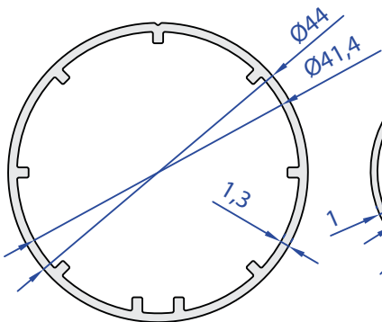
60091-00 0,538 kg/m
