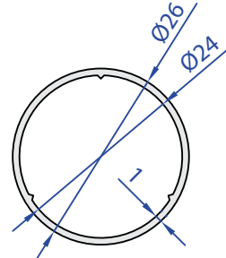
60014-00 0,215 kg/m
