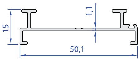
60425-00 0,308 Kg/m
