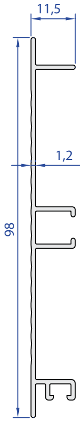
60356-00 0,465 Kg/m
