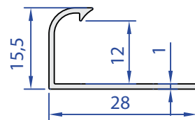
60072-00 0,132 kg/m
