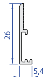
60045-00 0,117 kg/m
