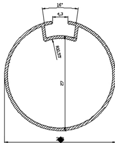
60794-00 0,233 Kg/m
