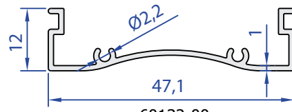
60132-00 0,238 kg/m
