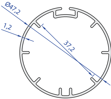
60424-00 0,594 Kg/m
