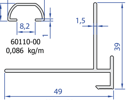
60054-00 0,397 kg/m
