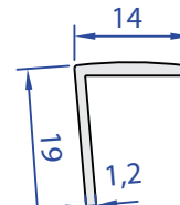
60020-00 0,113 kg/m
