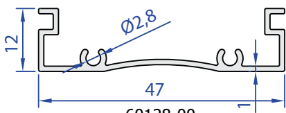
60128-00 0,260 kg/m
