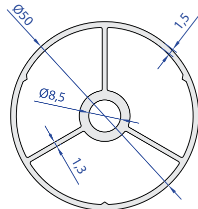
05916-00 1,038 Kg/m
