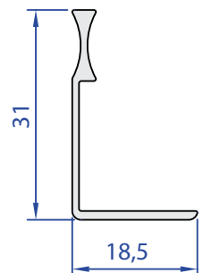
60431-00 0,170 Kg/m
