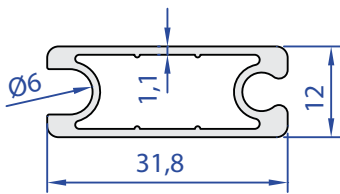
60107-00 0,334 kg/m
