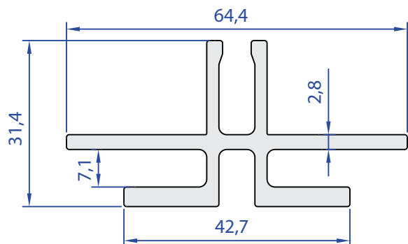
60126-00 1,181 kg/m
