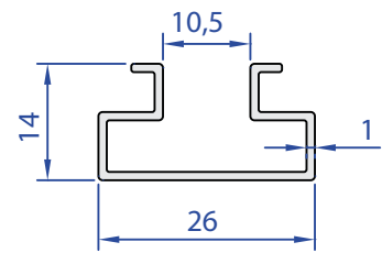
60451-00 0,192 Kg/m
