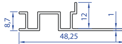
60075-00 0,239 kg/m
