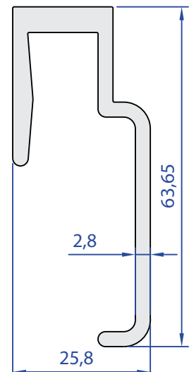
60113-00 0,992 kg/m
