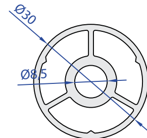
05915-00 0,677 Kg/m
