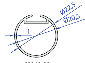
60040-00 0,212 kg/m
