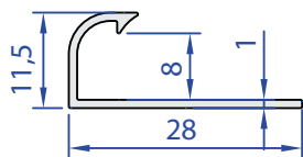
60032-00 0,121 kg/m
