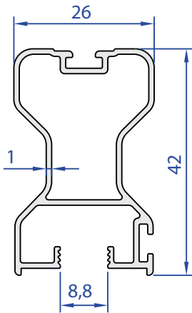
60442-00 0,455 Kg/m
