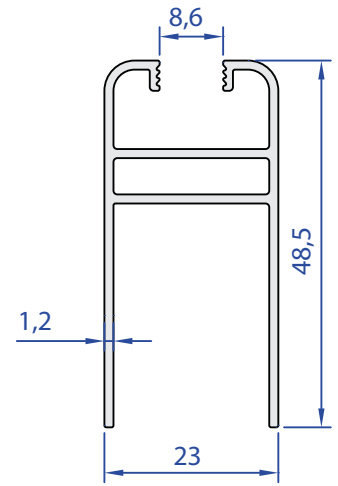
60177-00 0,496 kg/m
