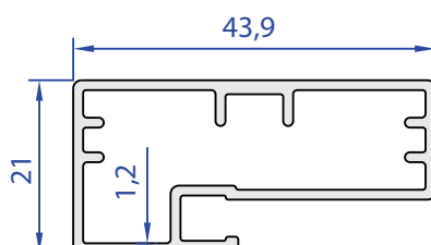
60274-00 0,506 Kg/m
