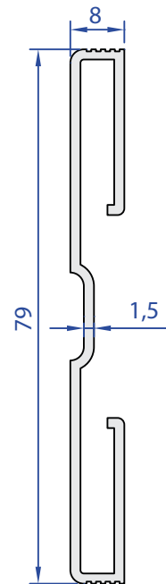
60007-00 0,567 kg/m
