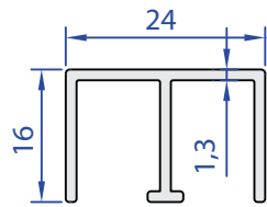
60136-00 0,250 kg/m
