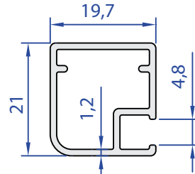
60277-00 0,282 Kg/m
