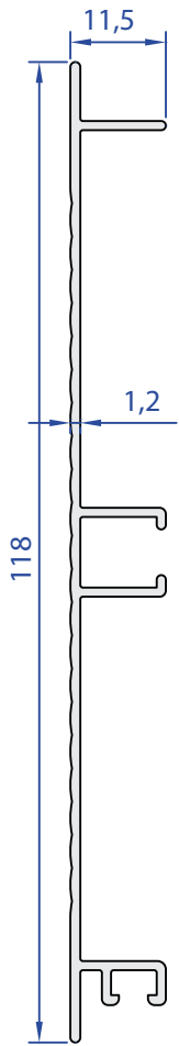
60357-00 0,527 Kg/m
