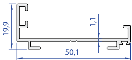
60146-00 0,306 Kg/m
