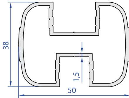
60043-00 0,910 kg/m
