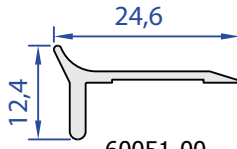
60051-00 0,129 kg/m
