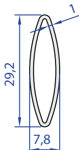
60026-00 0,162 kg/m
