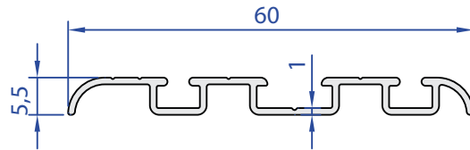
60390-00 0,270 Kg/m
