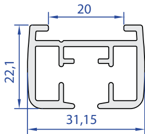
05074-00 0,545 kg/m
