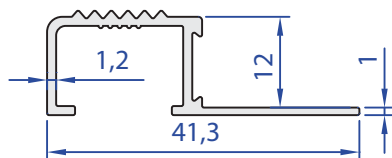
60086-00 0,236 kg/m
