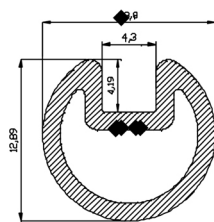
60796-00 0,176 Kg/m
