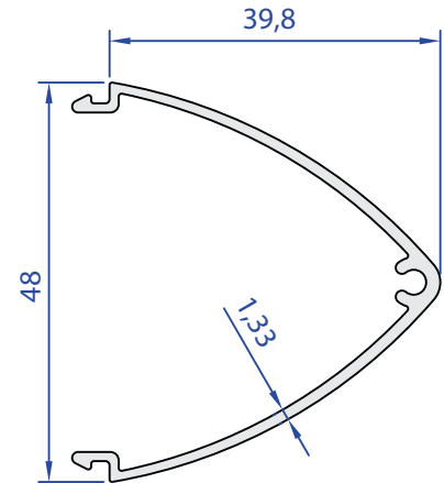
05914-00 0,405 Kg/m
