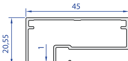
60433-00 0,390 Kg/m
