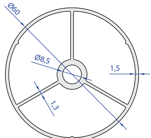
05917-00 1,219 Kg/m
