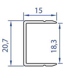
60210-00 0,151 Kg/m
