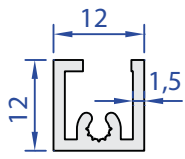
60011-00 0,174 kg/m
