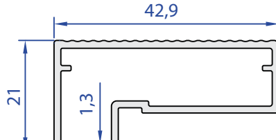
60450-00 0,477 Kg/m
