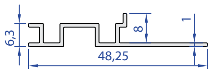
60073-00 0,209 kg/m
