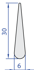
60015-00 0,292 kg/m
