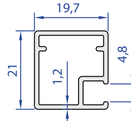
60276-00 0,286 Kg/m
