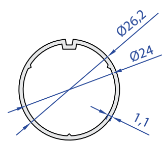
60094-00 0,244 kg/m
