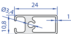
60087-00 0,253 kg/m
