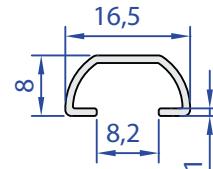
60110-00 0,086 kg/m
