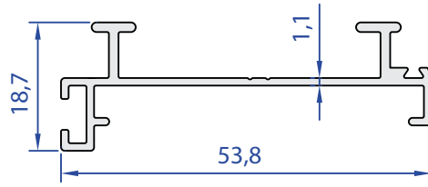
60423-00 0,352 Kg/m
