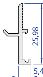
05051-00 0,164 kg/m
