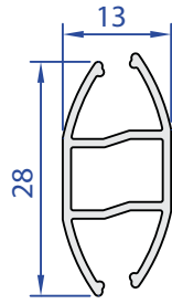
60105-00 0,226 kg/m
