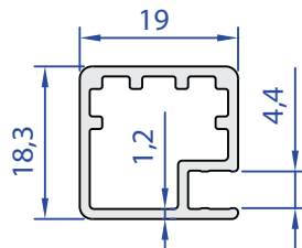
60394-00 0,280 Kg/m
