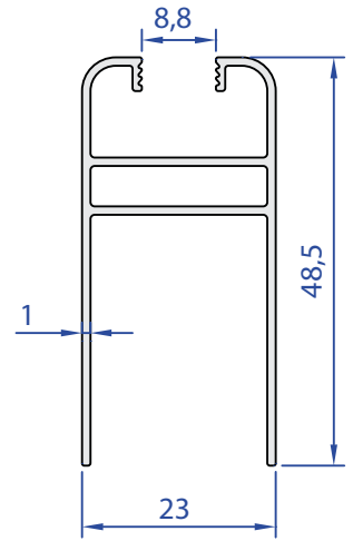
60441-00 0,417 Kg/m
