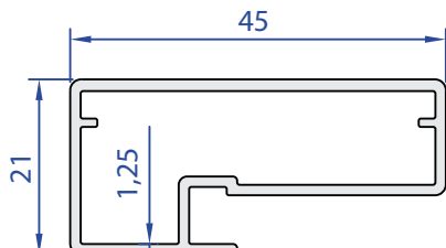
60224-00 0,480 Kg/m
