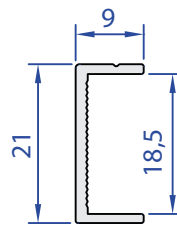
60364-00 0,138 Kg/m
