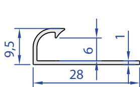
60071-00 0,116 kg/m
