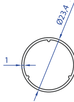
60459-00 0,280 Kg/m
