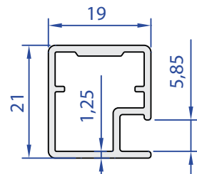
60211-00 0,300 Kg/m
