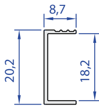
60173-00 0,091 kg/m
