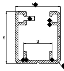
60797-00 0,215 Kg/m
