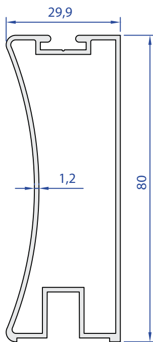
60006-00 0,827 kg/m
