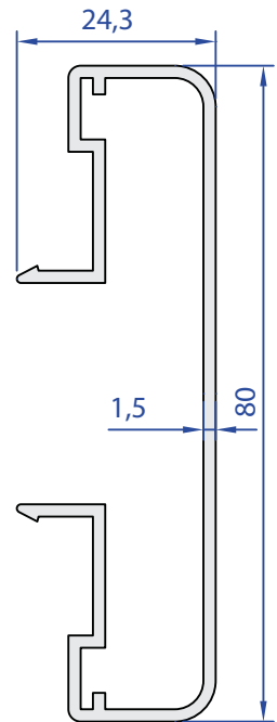
60009-00 0,761 kg/m
