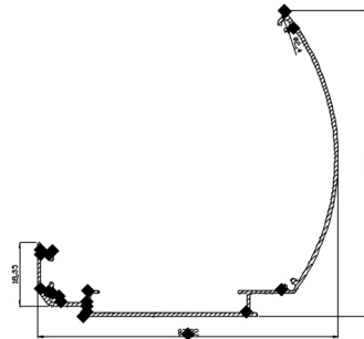
60792-00 0,584 Kg/m
