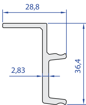
60572-00 0,438 Kg/m
