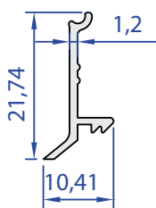
60052-00 0,099 kg/m
