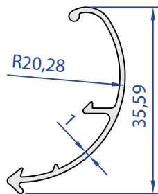
60053-00 0,183 kg/m
