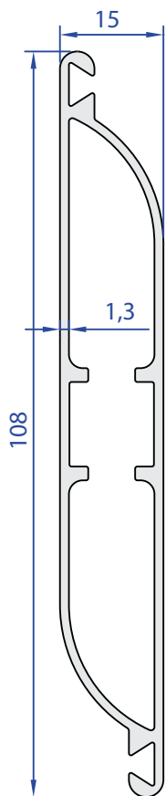
55489-00 0,888 Kg/m
