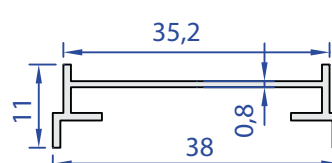
55046-00 0,162 kg/m
