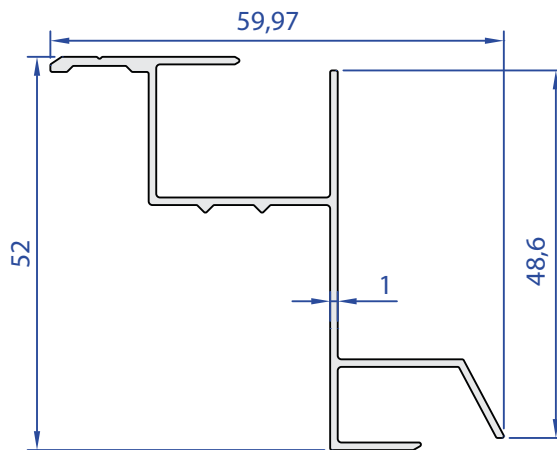
55485-00 0,443 Kg/m
