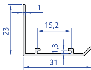
55347-00 0,169 kg/m
