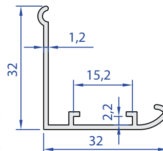
55065-00 0,256 kg/m
