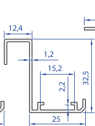
55191-00 0,296 kg/m
