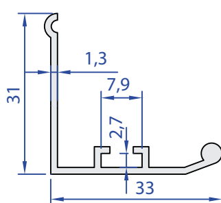
55013-00 0,289 kg/m
