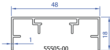
55505-00 0,309 Kg/m
