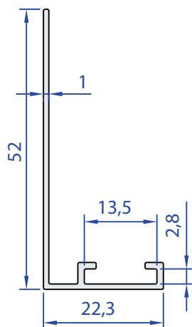
55561-00 0,239 Kg/m
