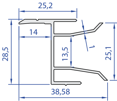
55253-00 0,348 kg/m
