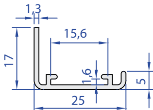
55093-00 0,179 kg/m
