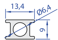
55674-00 0,163 Kg/m
