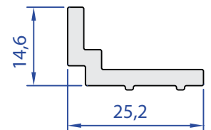
55447-00 0,298 Kg/m
