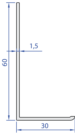
55430-00 0,360 Kg/m
