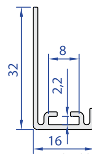
55184-00 0,201 kg/m
