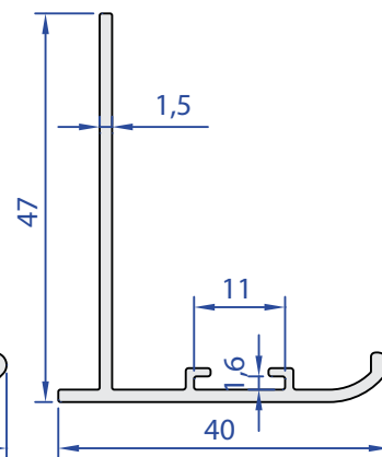
55547-00 0,384 Kg/m
