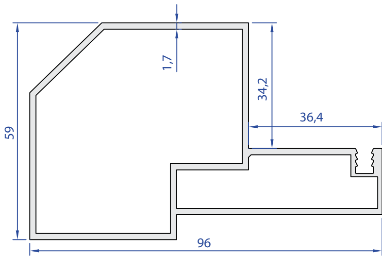
55406-00 1544,8 Kg/m
