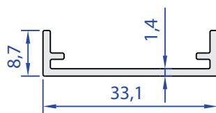
55467-00 0,198 Kg/m
