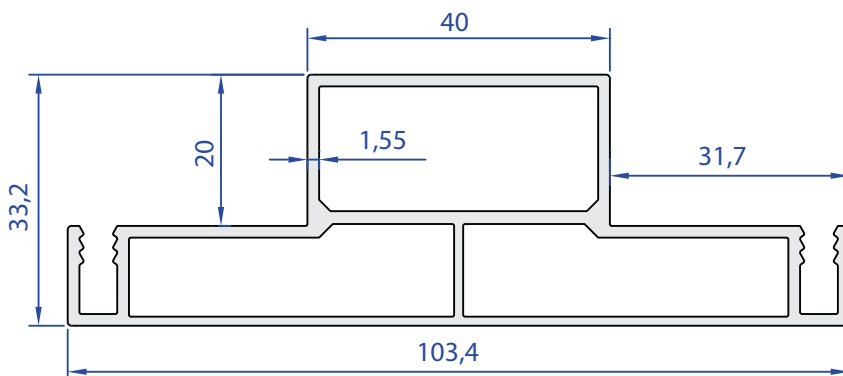
55401-00 1,321 Kg/m
