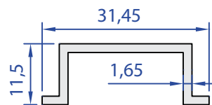
55607-00 0,228 Kg/m
