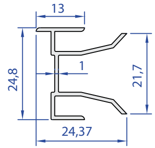
55152-00 0,230 kg/m
