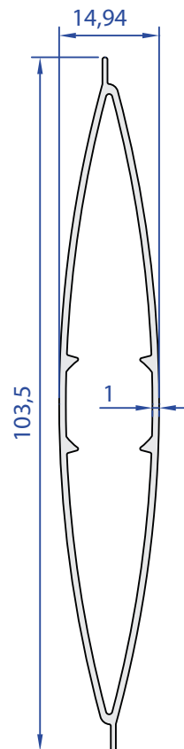
55396-00 0,566 Kg/m
