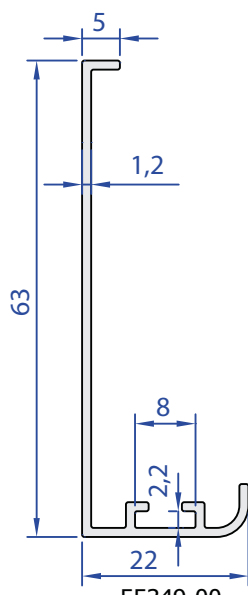
55349-00 0,332 kg/m
