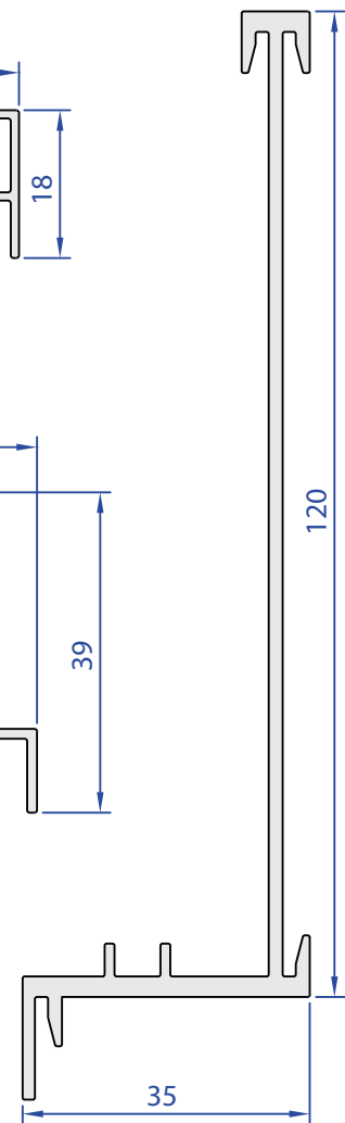
55391-00 0,979 Kg/m
