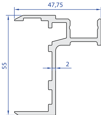
55316-00 0,877 Kg/m
