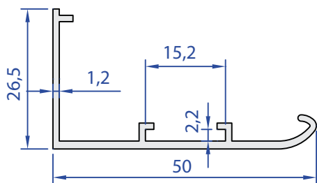
55069-00 0,337 kg/m
