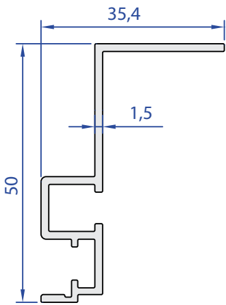
55281-00 0,441 kg/m
