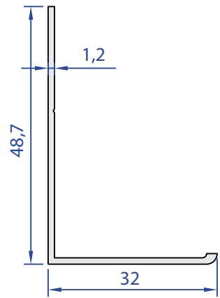
55517-00 0,261 Kg/m
