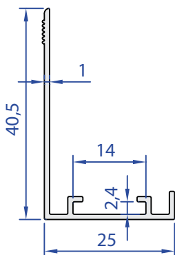
55744-00 0,218 Kg/m
