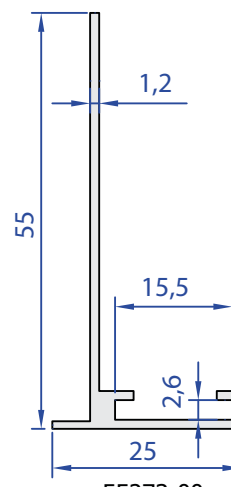
55273-00 0,302 kg/m
