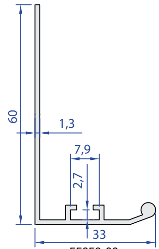
55059-00 0,388 kg/m
