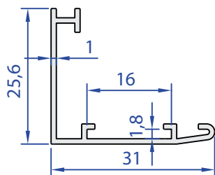
55078-00 0,204 kg/m
