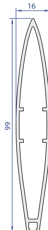
55679-00 0,849 Kg/m
