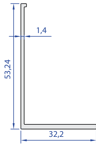
55539-00 0,373 Kg/m
