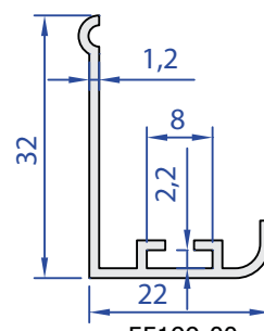
55199-00 0,226 kg/m
