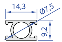
55529-00 0,144 Kg/m
