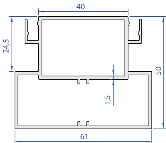
55283-00 1,114 kg/m
