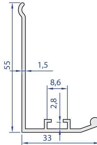
55016-00 0,415 kg/m
