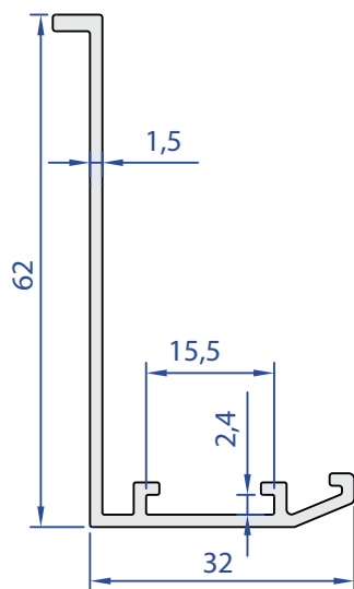
55677-00 0,462 Kg/m
