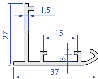
55027-00 0,330 kg/m
