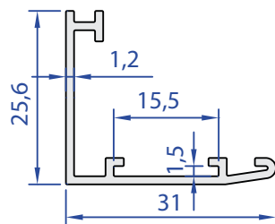
55116-00 0,242 kg/m
