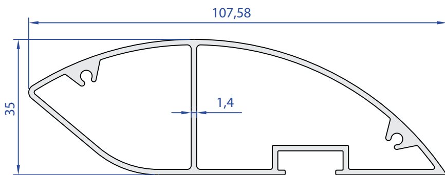
55331-00 1,197 Kg/m
