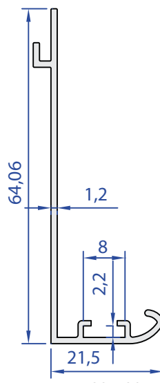
55224-00 0,336 kg/m
