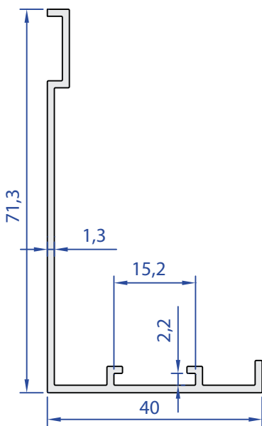
55088-00 0,479 kg/m
