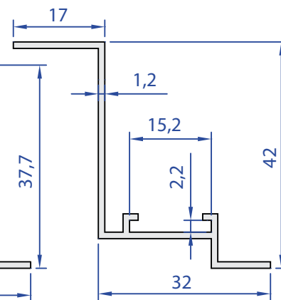
55160-00 0,321 kg/m
