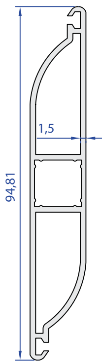
55056-00 0,875 Kg/m
