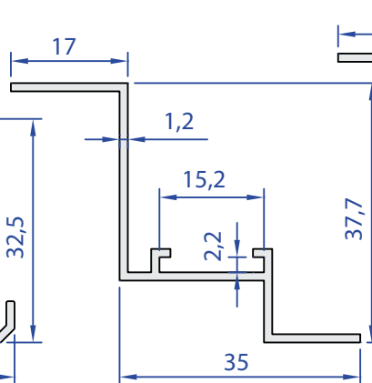
55166-00 0,317 kg/m
