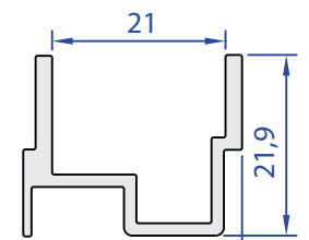
55279-00 0,334 kg/m
