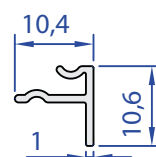
55278-00 0,065 kg/m
