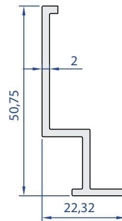
55790-00 0,405 Kg/m
