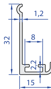
55483-00 0,198 Kg/m
