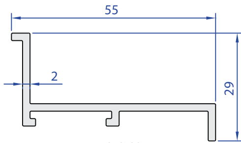
55670-00 0,504 Kg/m
