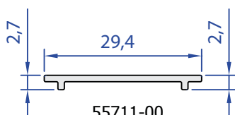
55711-00 0,105 Kg/m
