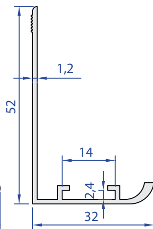
55503-00 0,329 Kg/m
