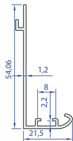
55150-00 0,303 kg/m
