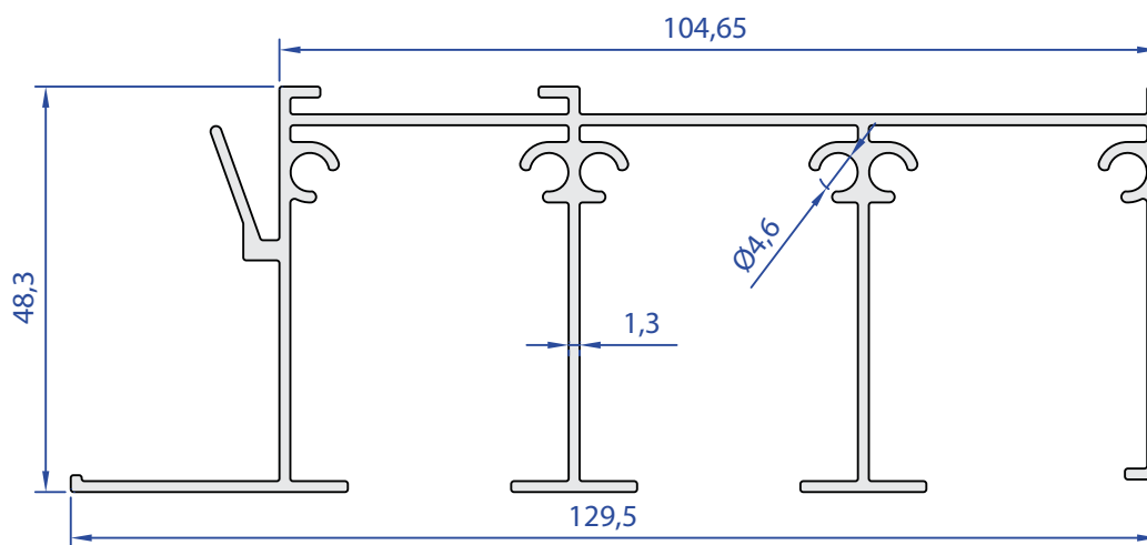
55651-00 1,579 Kg/m
