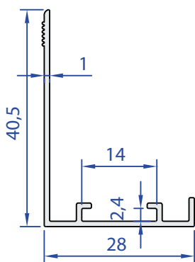
55734-00 0,227 Kg/m
