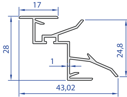
55175-00 0,336 kg/m
