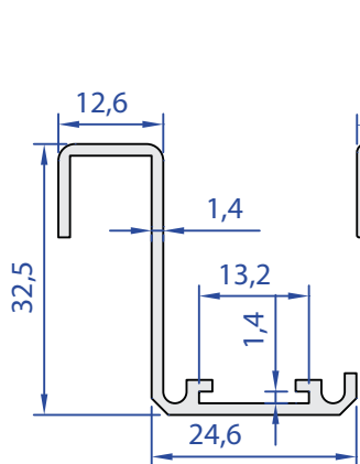
55070-00 0,328 kg/m
