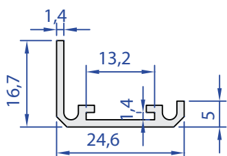
55019-00 0,194 kg/m
