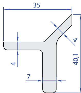
55285-00 0,887 kg/m
