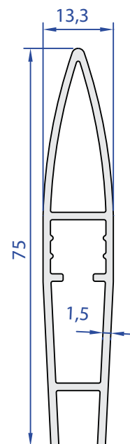
55533-00 0,680 Kg/m
