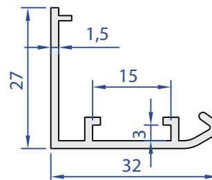
55025-00 0,306 kg/m
