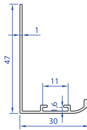
55545-00 0,244 Kg/m
