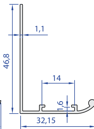
55394-00 0,271 Kg/m
