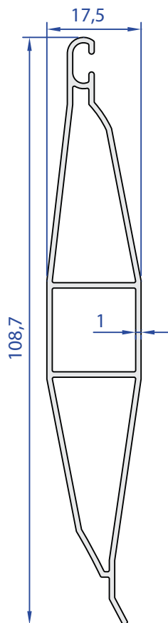
55480-00 0,666 Kg/m
