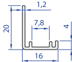
55213-00 0,136 kg/m
