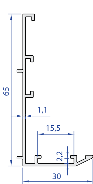
55378-00 0,383 Kg/m
