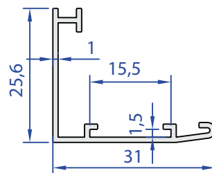
55086-00 0,203 kg/m
