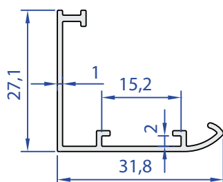
55100-00 0,210 kg/m
