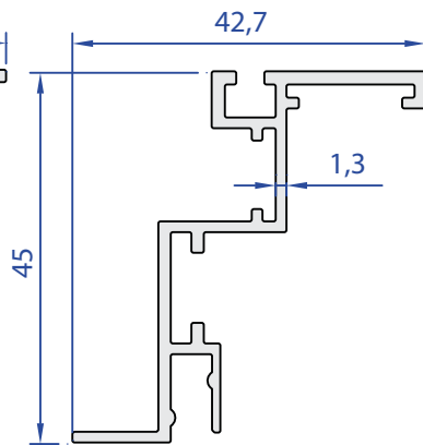
55282-00 0,499 kg/m
