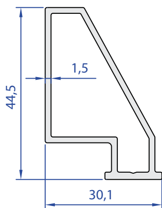
55380-00 0,540 Kg/m
