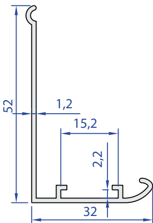
55064-00 0,321 kg/m
