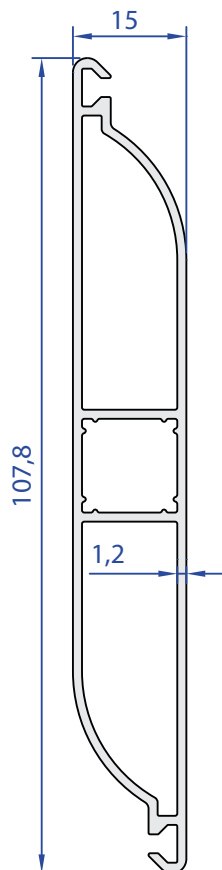
55455-00 0,821 Kg/m
