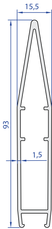
55550-00 0,835 Kg/m
