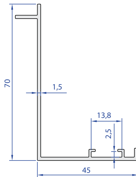
55486-00 0,547 Kg/m
