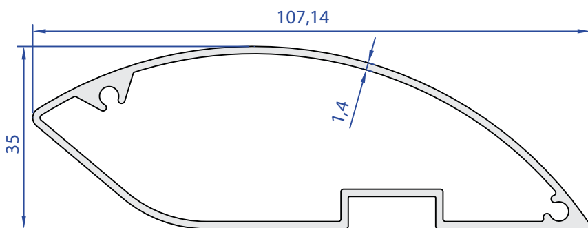
55553-00 1,034 Kg/m
