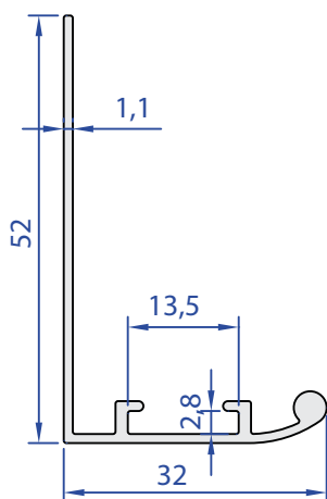
55496-00 0,320 Kg/m
