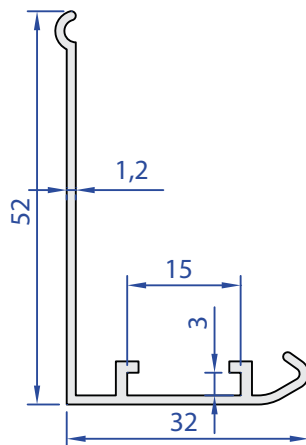
55050-00 0,337 kg/m
