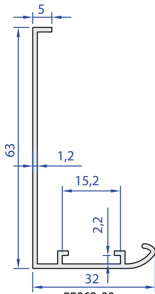
55063-00 0,365 kg/m
