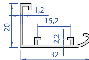
55072-00 0,231 kg/m
