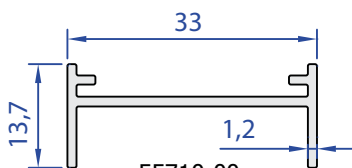
55710-00 0,213 Kg/m
