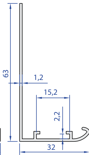
55190-00 0,352 kg/m
