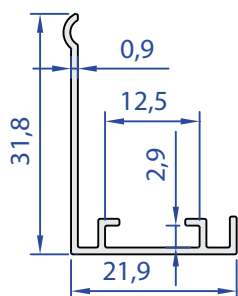
55212-00 0,168 kg/m
