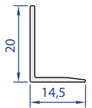
55655-00 0,104 Kg/m
