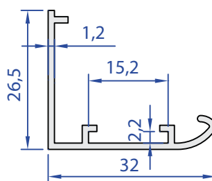
55066-00 0,242 kg/m
