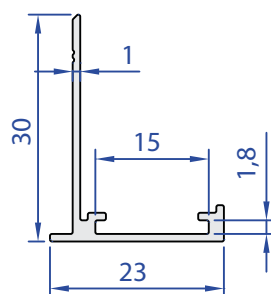
55524-00 0,178 Kg/m
