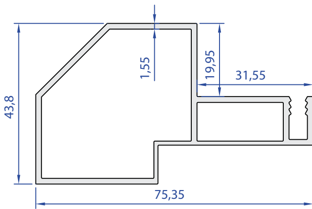
55399-00 0,950 Kg/m
