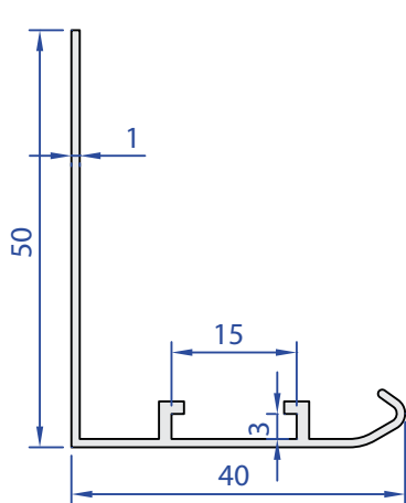
55530-00 0,303 Kg/m
