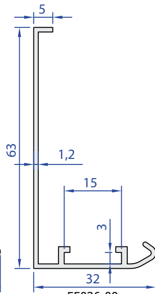
55026-00 0,381 kg/m
