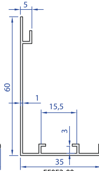
55052-00 0,321 kg/m
