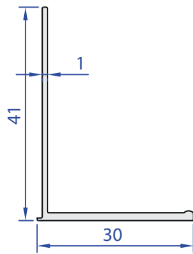
55782-00 0,228 Kg/m
