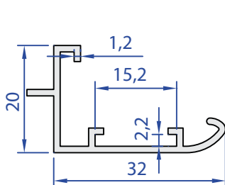
55075-00 0,247 kg/m
