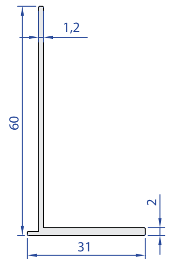
55250-00 0,348 kg/m
