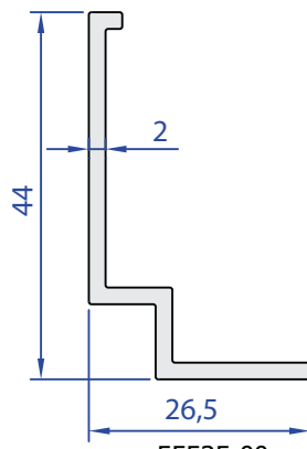
55535-00 0,382 Kg/m
