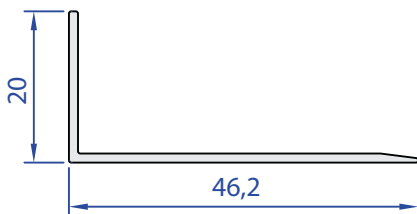
55654-00 0,207 Kg/m
