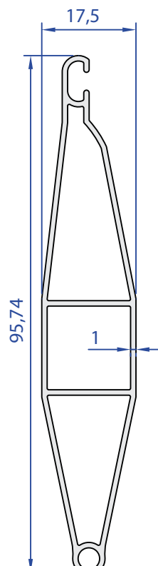
55683-00 0,629 Kg/m
