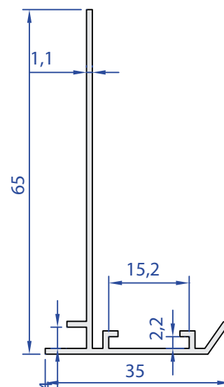
55328-00 0,343 kg/m
