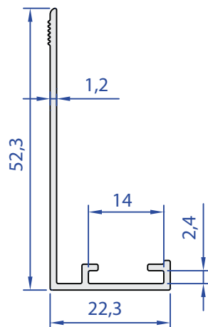
55555-00 0,282 Kg/m
