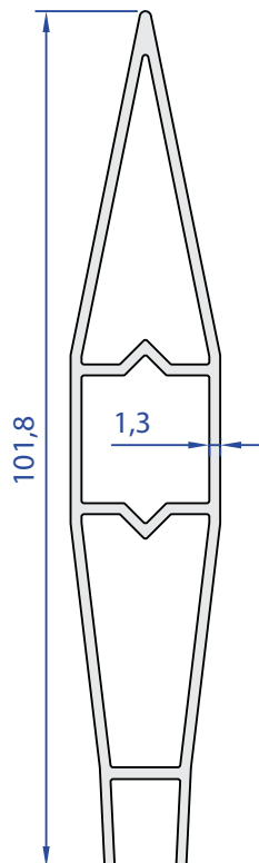
55574-00 0,867 Kg/m
