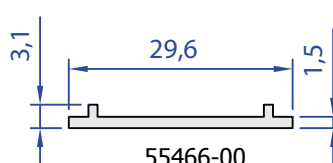
55466-00 0,131 Kg/m
