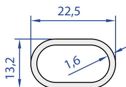
40193-00 0,239 Kg/m
