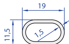
40194-00 0,189 Kg/m
