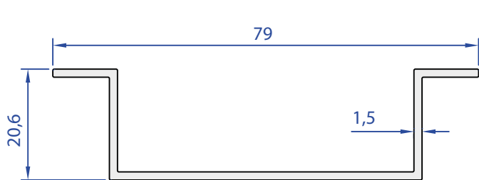
40131-00 0,477 Kg/m
