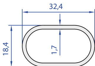
40191-00 0,370 Kg/m
