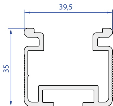
40210-00 0,792 Kg/m
