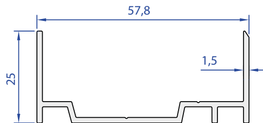
40130-00 0,462 Kg/m
