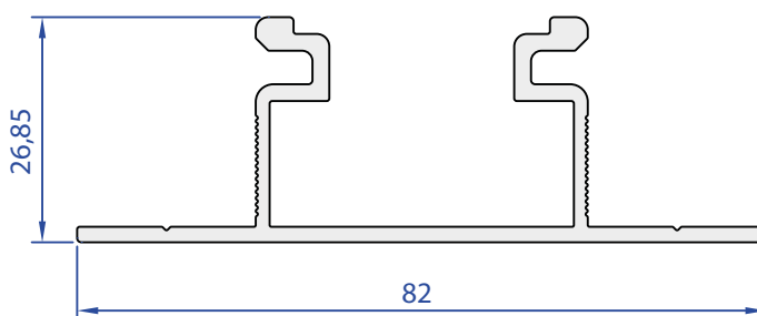
40209-00 0,803 Kg/m
