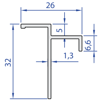
05234-00 0,221 kg/m
