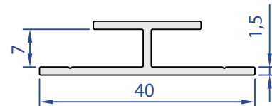
50032-00 0,272 Kg/m
