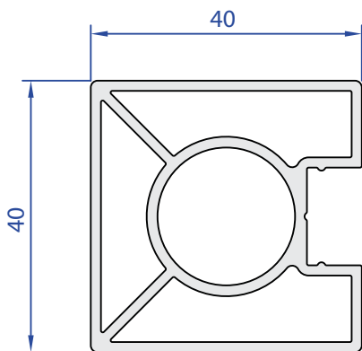
50141-00 1,080 Kg/m
