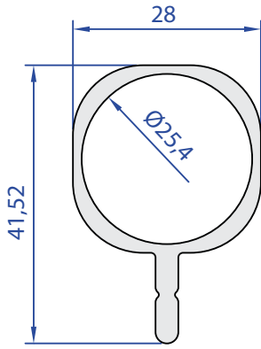
50041-00 0,615 Kg/m
