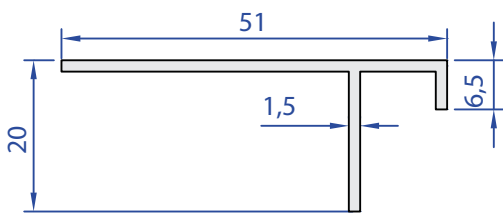
05504-00 0,303 kg/m
