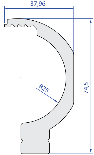
50043-00 2,072 Kg/m
