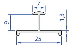
05430-00 0,147 kg/m
