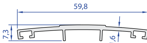
05237-00 0,345 kg/m
