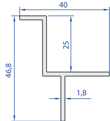
05581-00 0,414 kg/m
