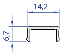
50137-00 0,078 Kg/m
