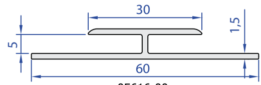
05616-00 0,382 kg/m
