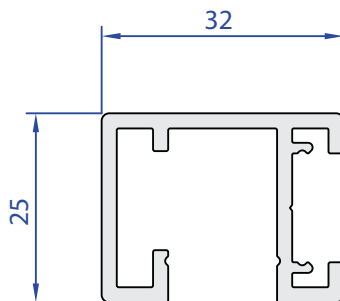
50140-00 0,588 Kg/m
