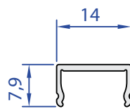
50136-00 0,079 Kg/m
