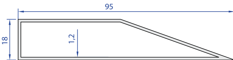
05137-00 0,656 kg/m
