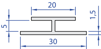
05083-00 0,224 kg/m
