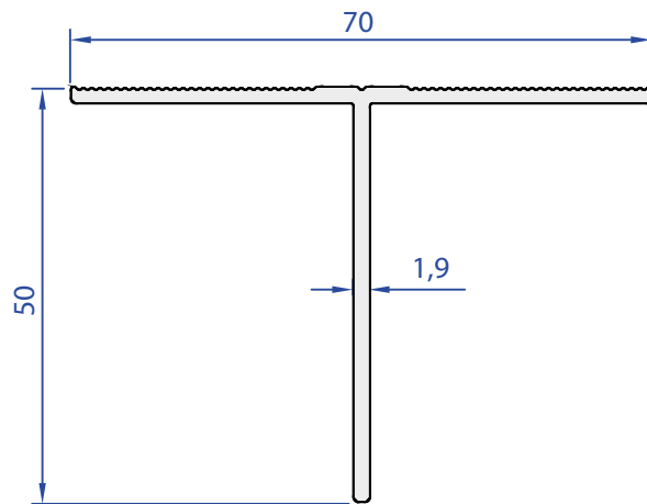
05280-00 0,568 kg/m
