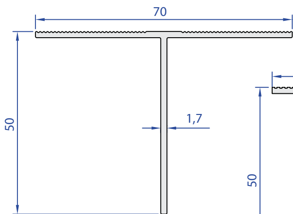
06286-00 0,518 Kg/m
